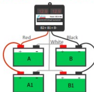
рис. 3 Банк батарей на 36В из 3-х АКБ
