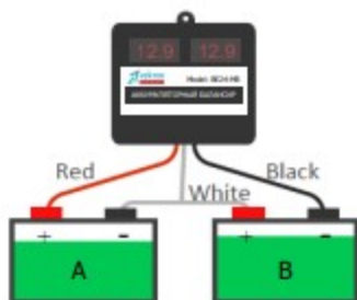
рис. 1 Банк батарей на 24В из 2-х АКБ
